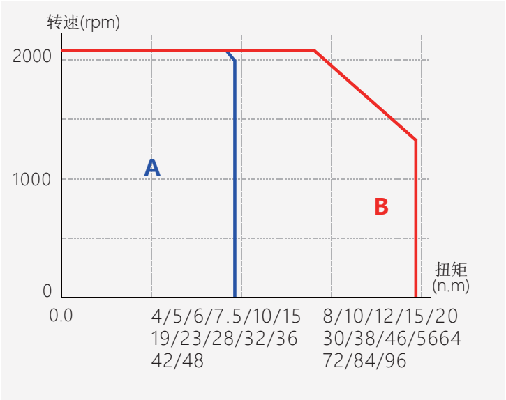
B:瞬时使用区域/Intermittent Duty Zoue
